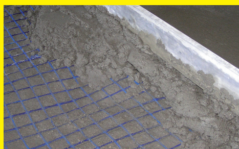
5. síť musí mít krytí min. 2 cm
