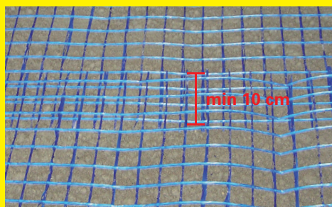
3. přesah sítí přes sebe min 10 cm
